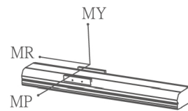
水平使用時 Static Loading Moment (單位:N.m)
